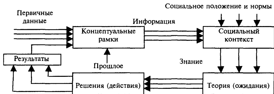
Рис. 8. Система «данные—информация—знания»
