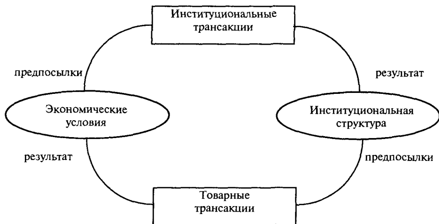
Рис. 14. Товарные и институциональные транзакции: кольцевая диаграмма
